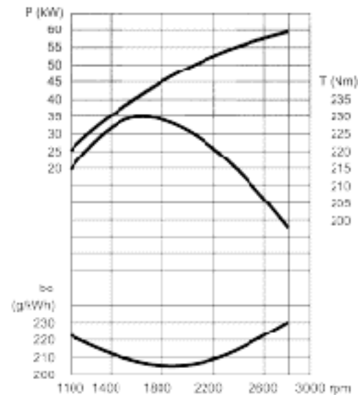
► BF4L2011
